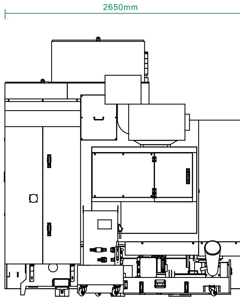
侧视图
