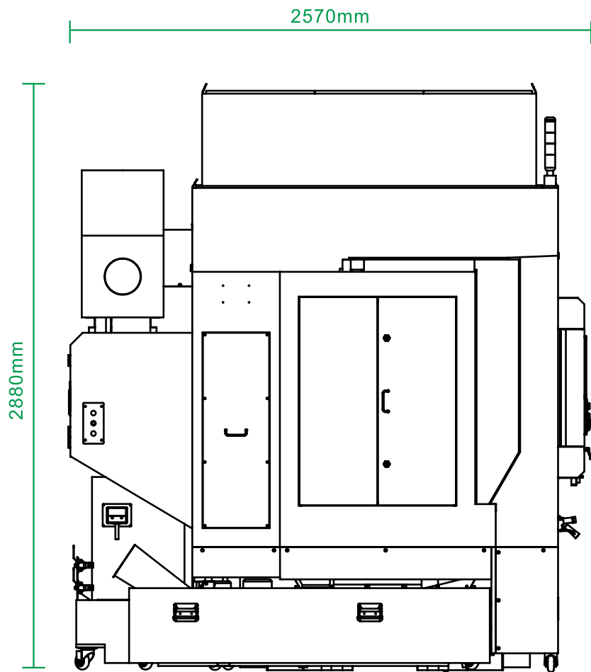
前视图
